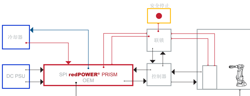
redPOWER® PRISM 原理图
